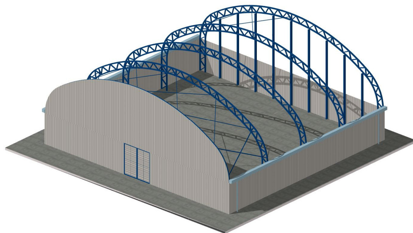
SPACCATO
