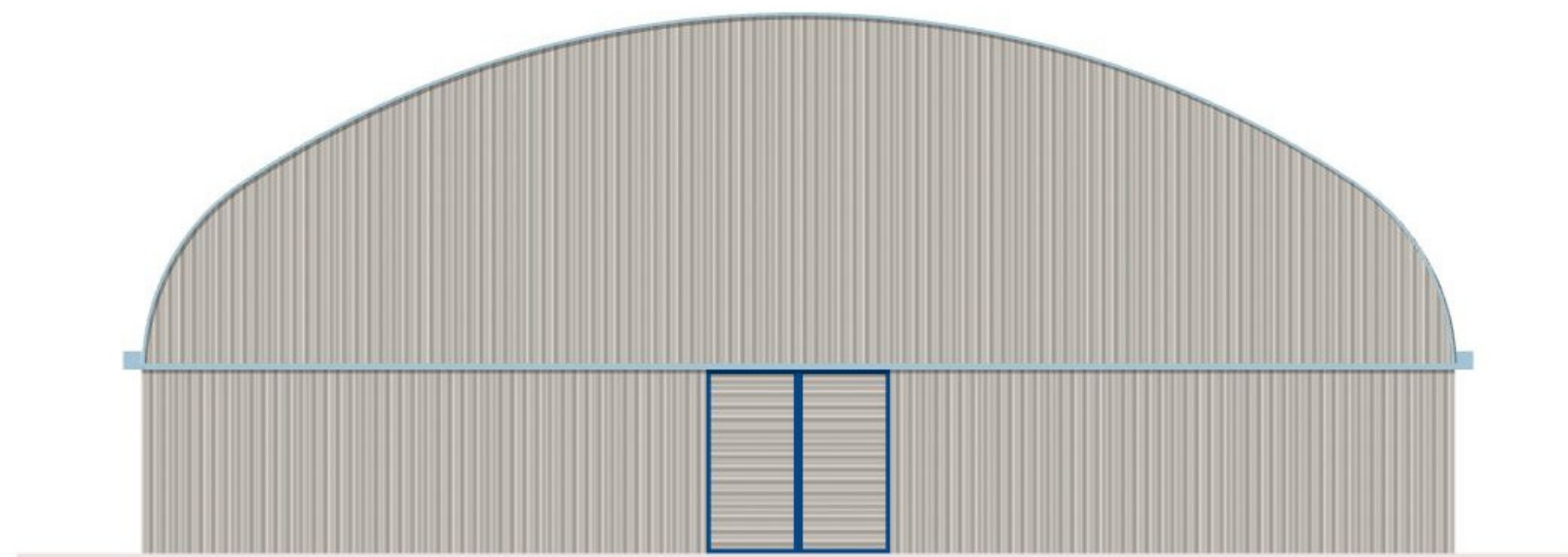
PROSPETTO FRONTALE scala 1/100
